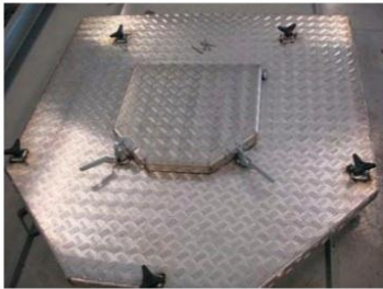
Silo lucka konstruerad för både bulkning, storsäcktömmning och fabriks-påfyllning.
